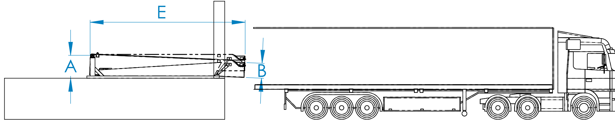
TELESKOBİK KONVEYÖR TAM KAPALI GÖRÜNÜŞ
